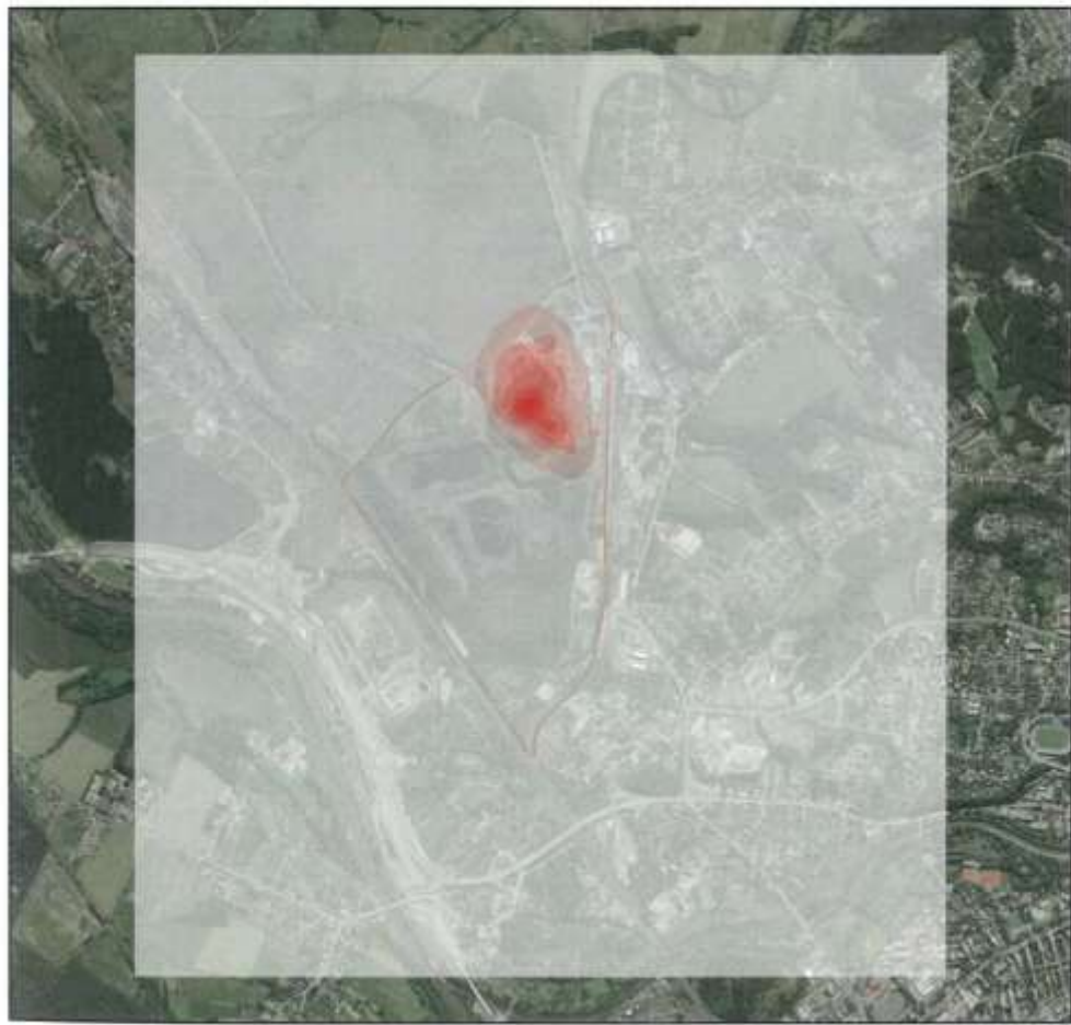
Roční průměrné koncentrace
