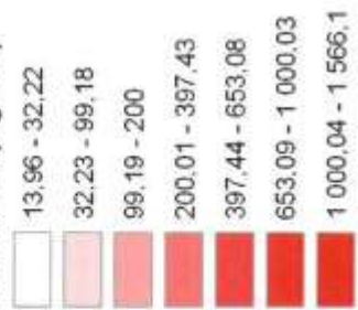
MAX NO2 (ug/m3)
