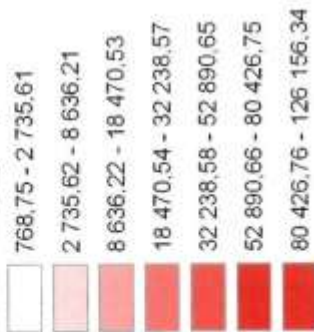
MAX CO (µg/m 3 )
