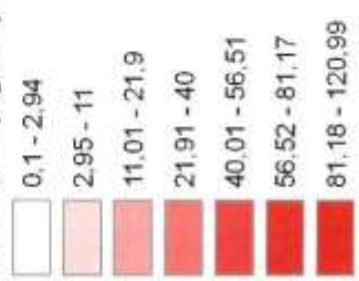
AVG NO2 (ug/m3)
